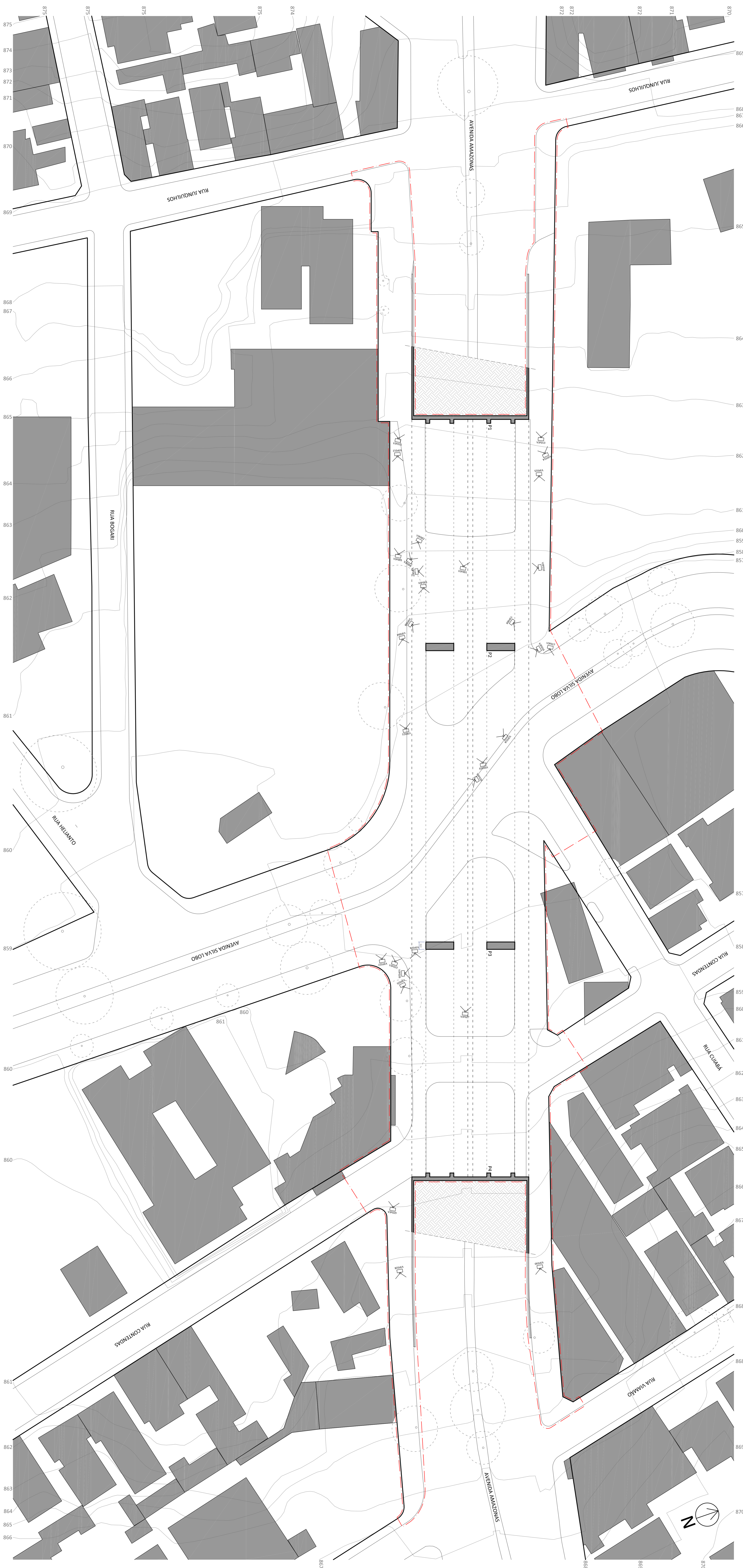
VIADUTO 3 | CINQUENTA E DOIS - AMAZONAS SOBRE SILVA LOBO BARRIOS PRADO, NOVA SUÍSSA E ALTO BARROCA - REGIONAL OESTE PLANTA GERAL | ESCALA: 1:500
